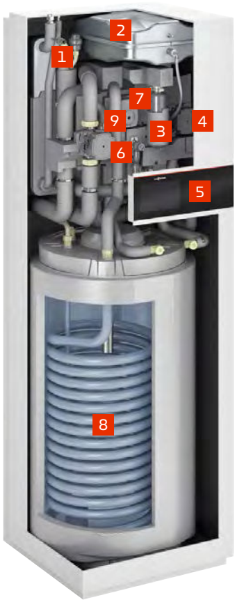
VITOCAL 222-S 2 integrierte Heiz-/Kühlkreise
